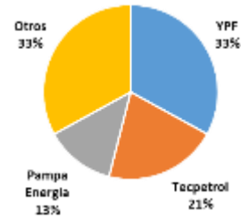
Gas no convencional Argentina (mcm/d. 2022)
