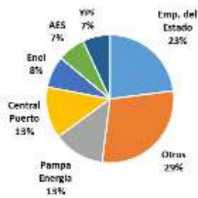
Generación eléctrica Argentina (% MW/tot. 2022)
